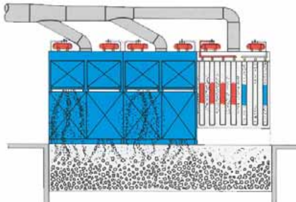
Construction Modulaire d'un mur d'aspiration sur fosse
